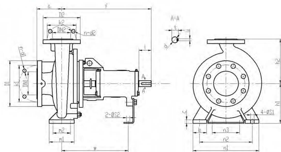
Монтажные размеры
