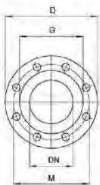
PN16 фланцы
