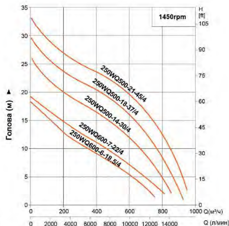
Производительность Q ►
