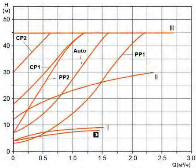
ARPXX-60 Q-P1
