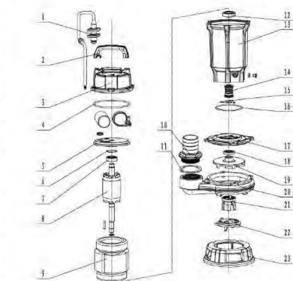
0,75-1,1 кВт Резьбовое соединение
