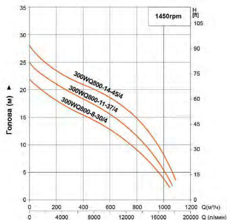
Производительность Q ►
